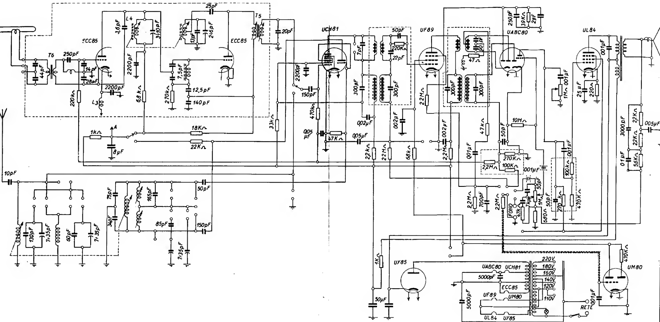
TELEFUNKEN RADIO TV - Apparecchi modd. MIGNONETTE MF prima serie e DOMINO terza serie. Sintonia a permeabilità variabile. Onde medie e corte a 25 e a 50 metri. Onde corte a modulazione di frequenza. Medie frequenze a 468 kc/s e a 10,7 Mc/s. Potenza d'uscita 4 watt.
